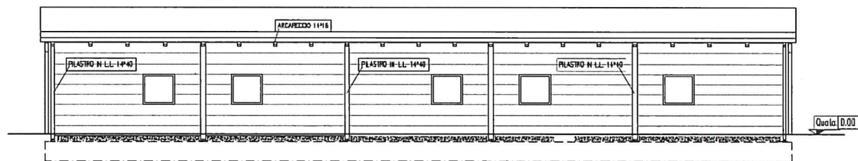
PROSPETTO NORD
