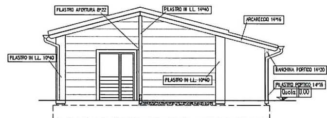
PROSPETTO OVEST
