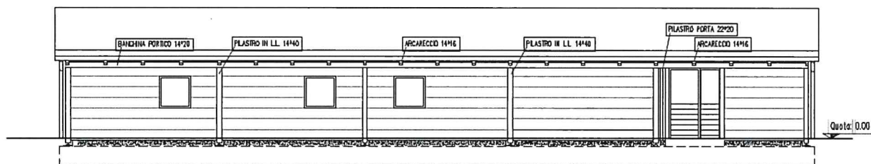
PROSPETTO SUD
