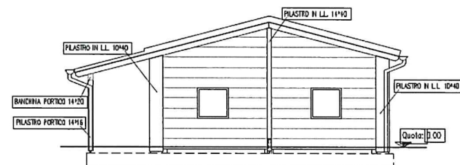
PROSPETTO EST
